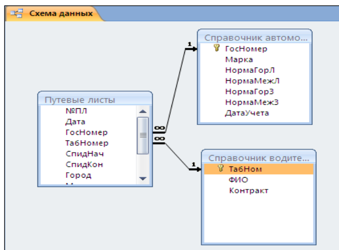
Рисунок 9 – Схема данных
